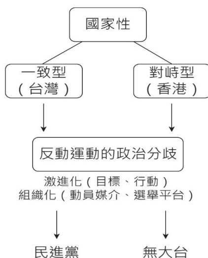
圖 2 研究架構圖
